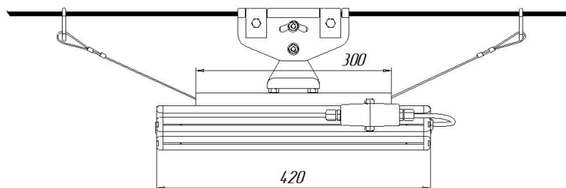
Светильник УСС 60 МАГИСТРАЛЬ Ш крепление на трос
