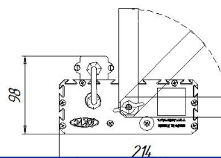
Светильник УСС 60 МАГИСТРАЛЬ Ш с креплением скоба
