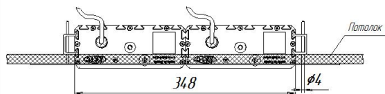
Светильник УСС 84 АЗС с 2Ех маркировкой; рамочное крепление
